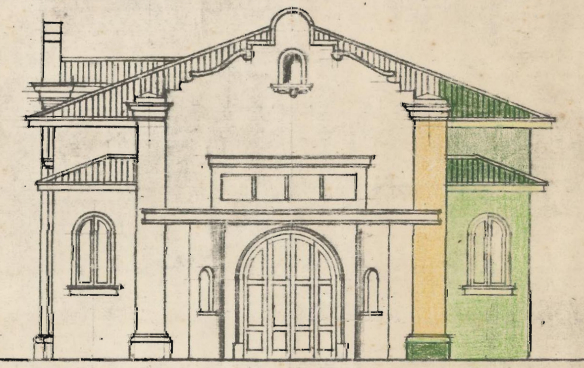
FACHADA SUR
