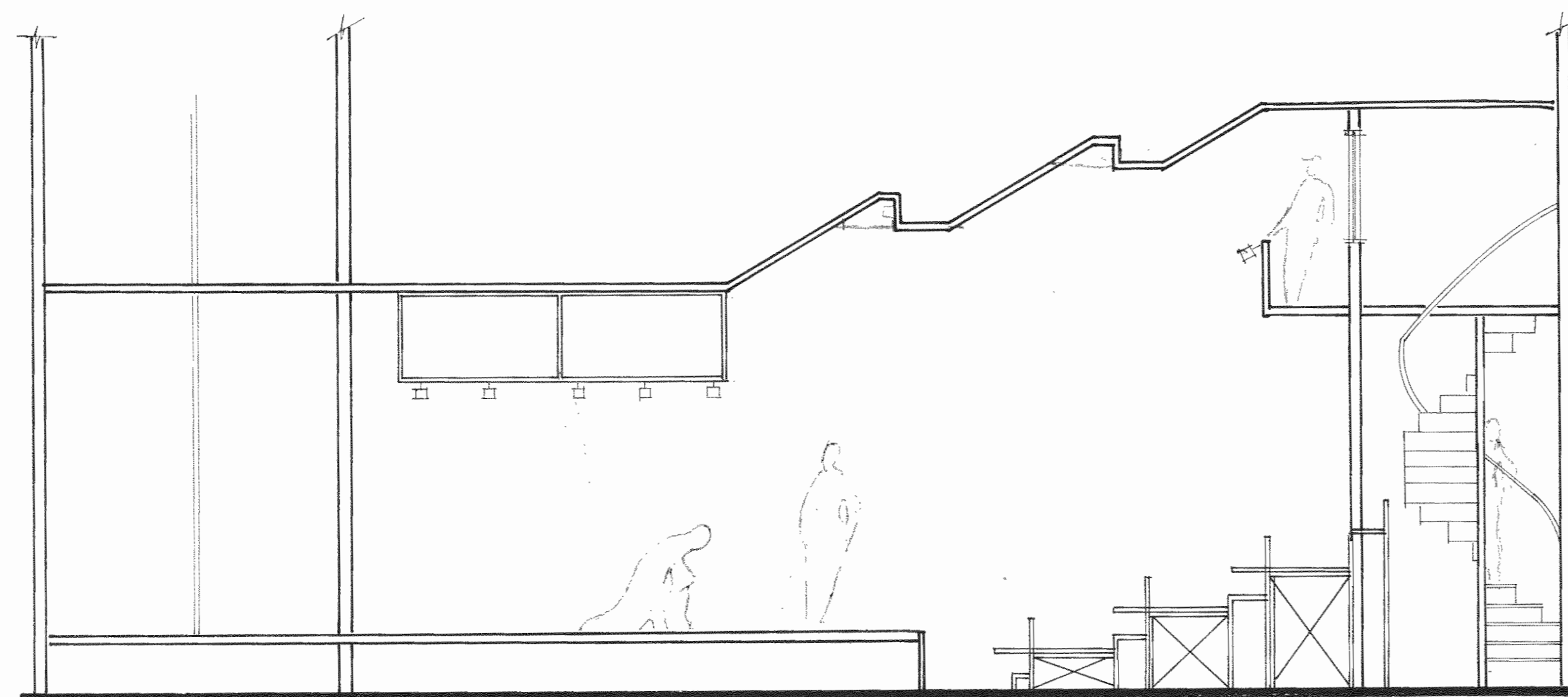
CORTE TRANSVERSAL B-B ESC. 1:50
