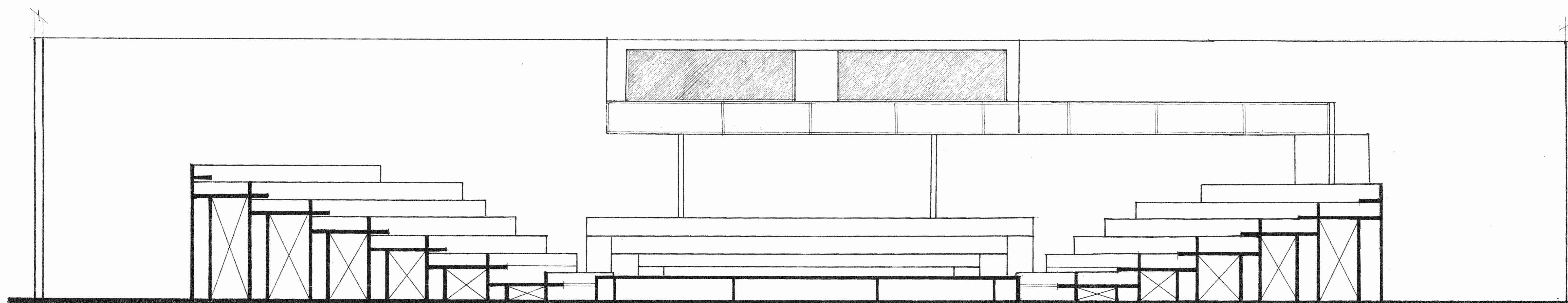
CORTE LONGITUDINAL A-A ESC. 1:50
