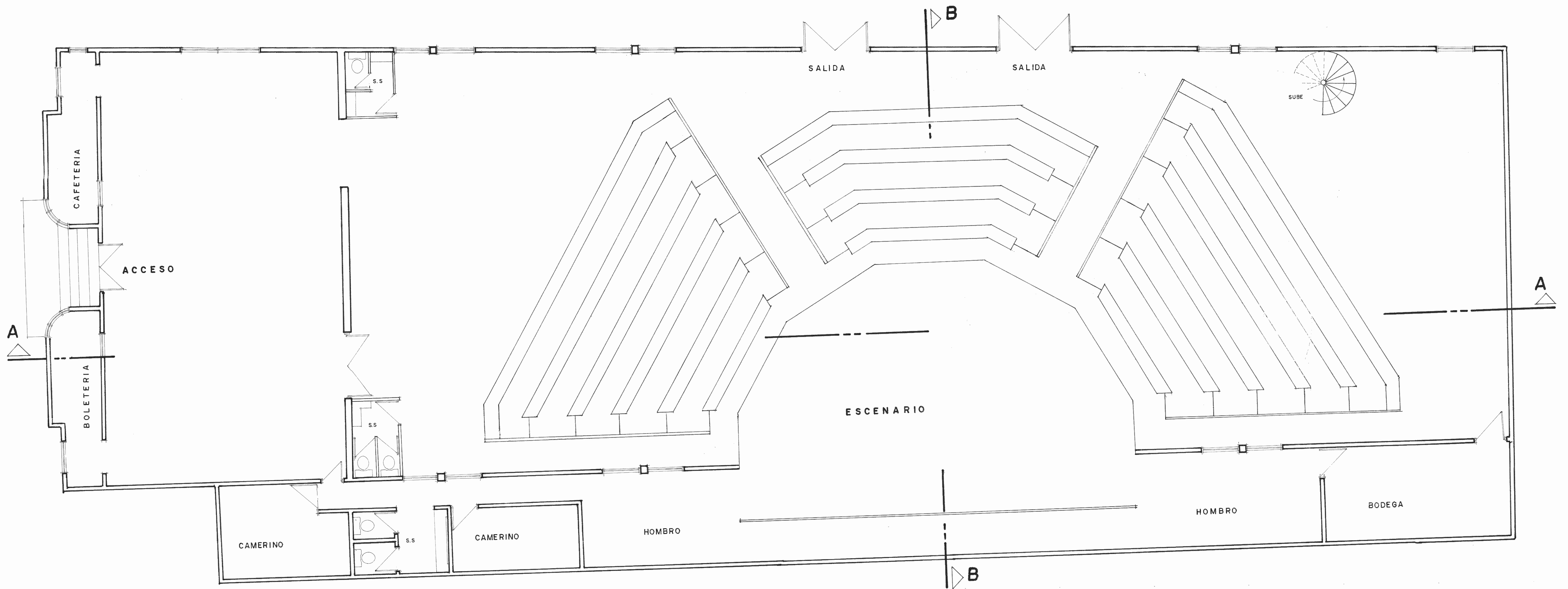
PLANTA DISTRIBUCION ARQUITECTONICA ESCALA 1:50
