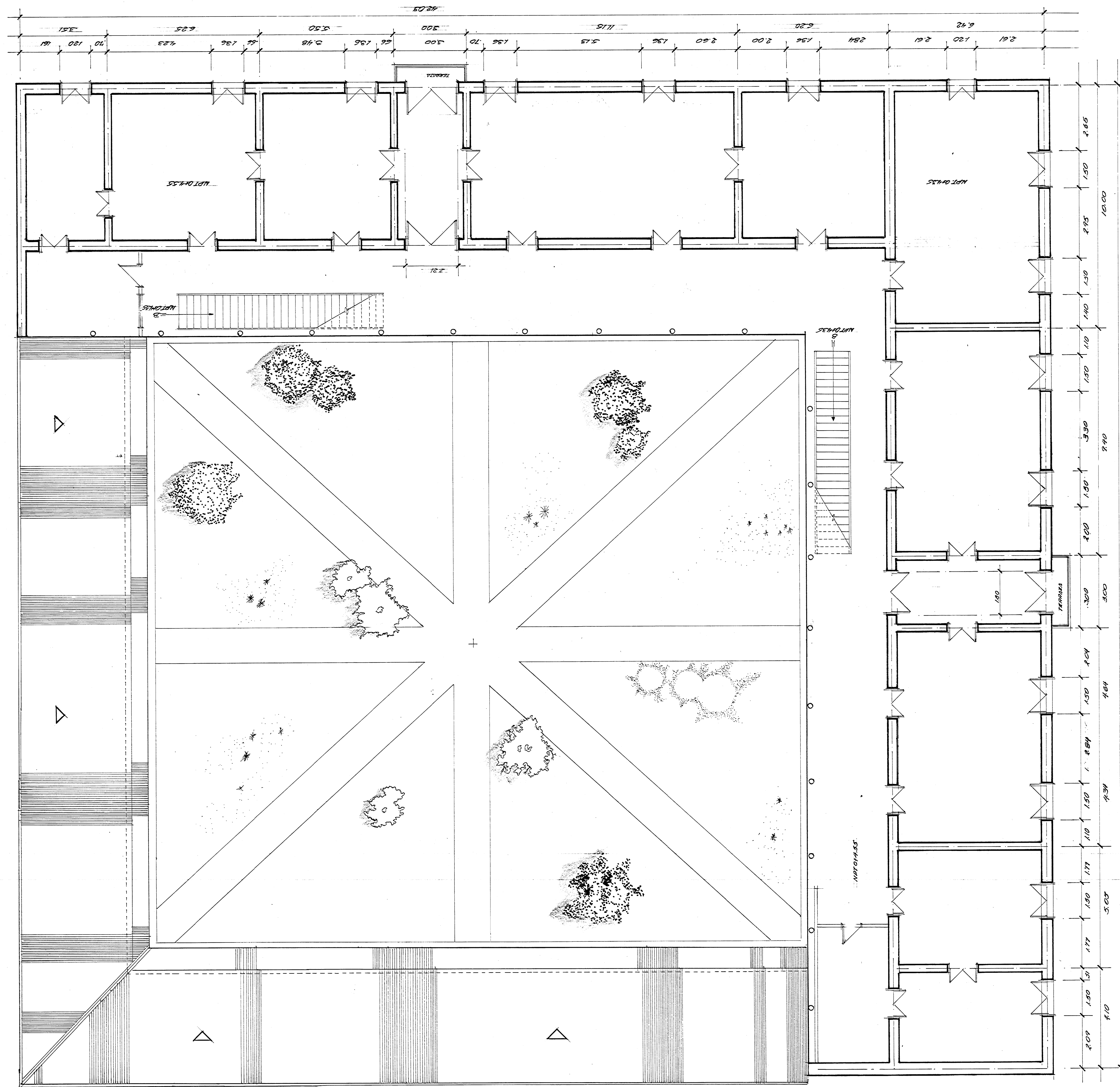
PLANTA ALTA DE DISTRIBUCION ARQUITECTONICA Esc. 1:75
